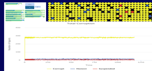
Imagen 2. Modelo de simulación de la corrupción con interacciones repetidas
